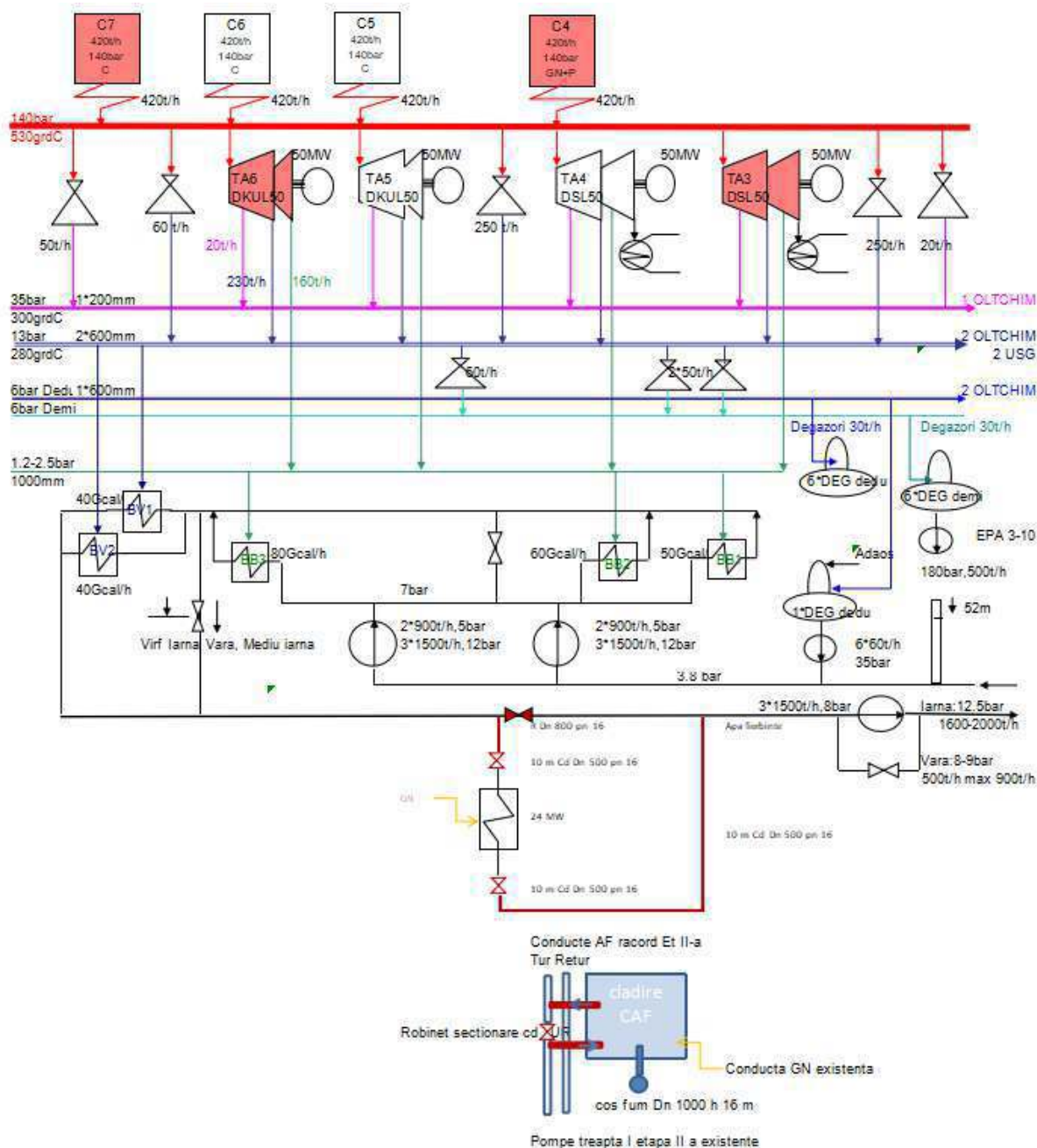
Figura 30. Schema de funcționare CET Govora 2022
