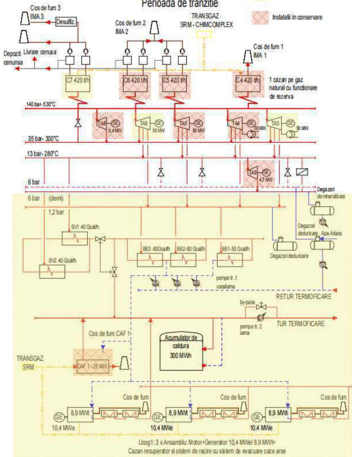
Figura 13. Schema simplificată CET Govora- situația propusă 2023
