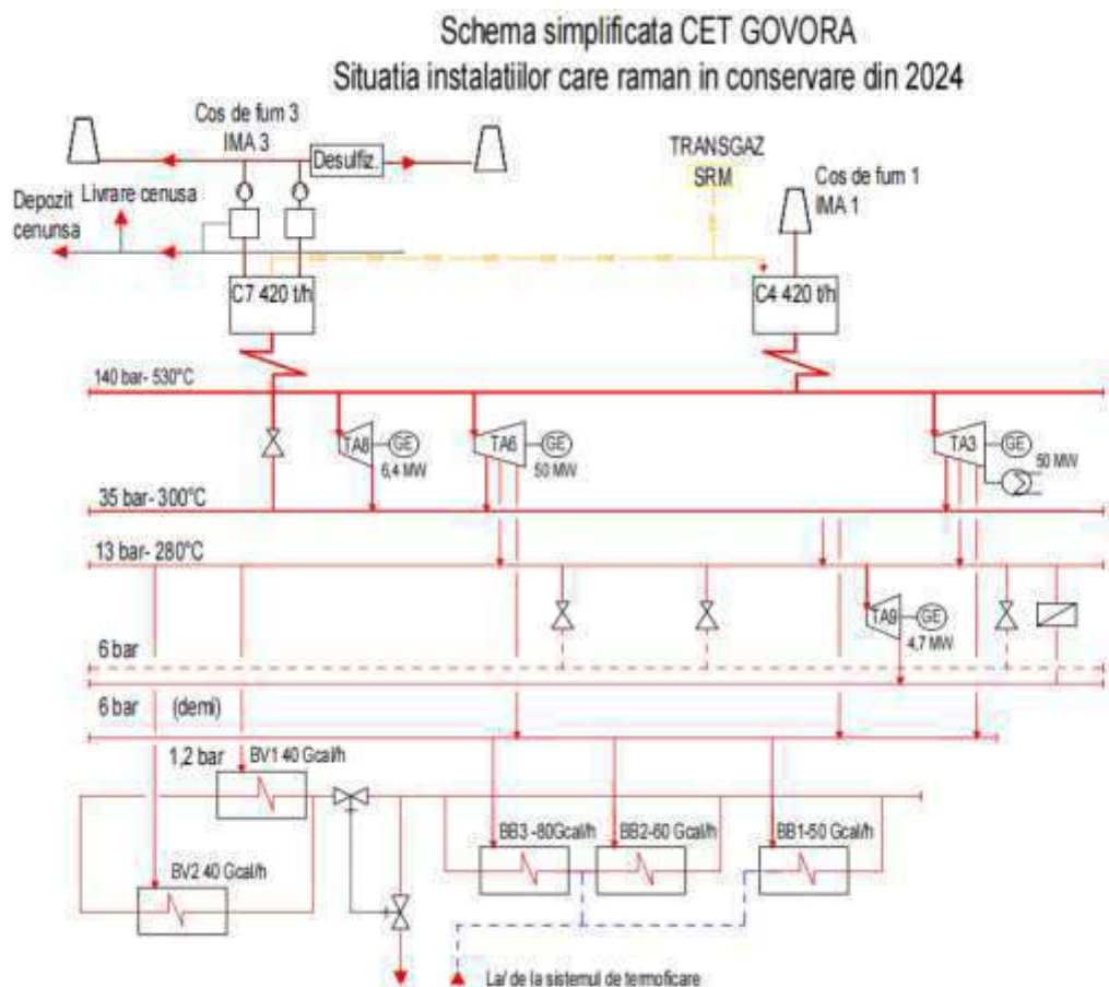
Figura 34. Schema instalațiilor ce intră în conservare din 2024
